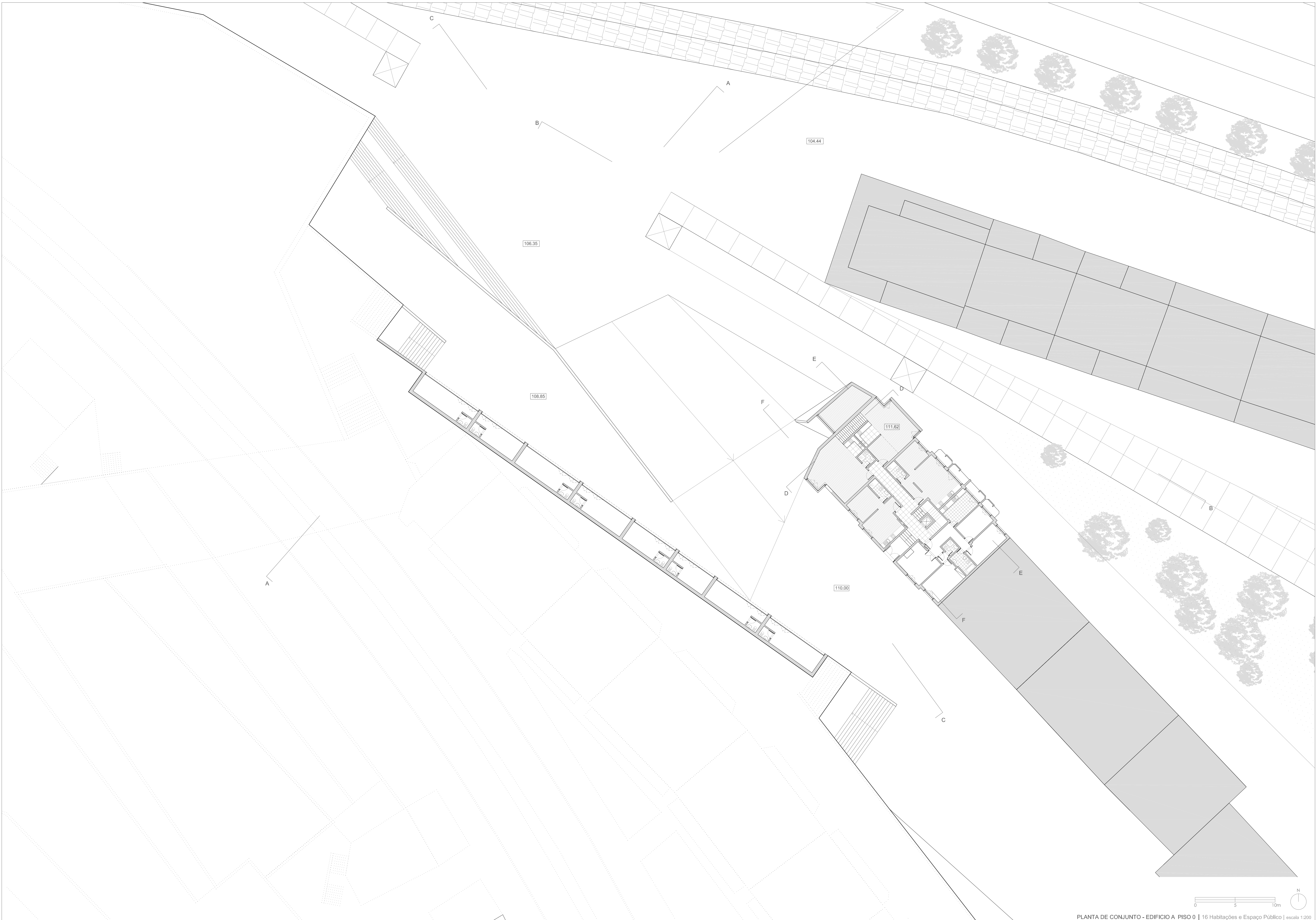
PLANTA DE CONJUNTO - EDIFÍCIO A PISO 0 | 16 Habitações e Espaço Público | escala 1:200 MIA, ISOTE 100, SUSANA ANASTÁCIO e 25045
