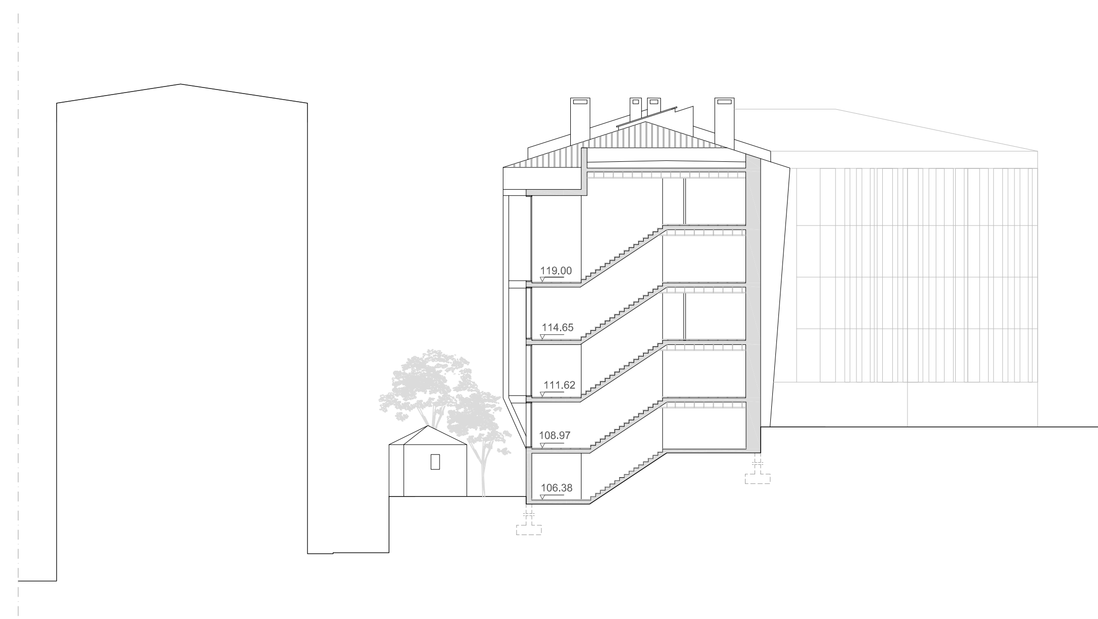
Corte DD
